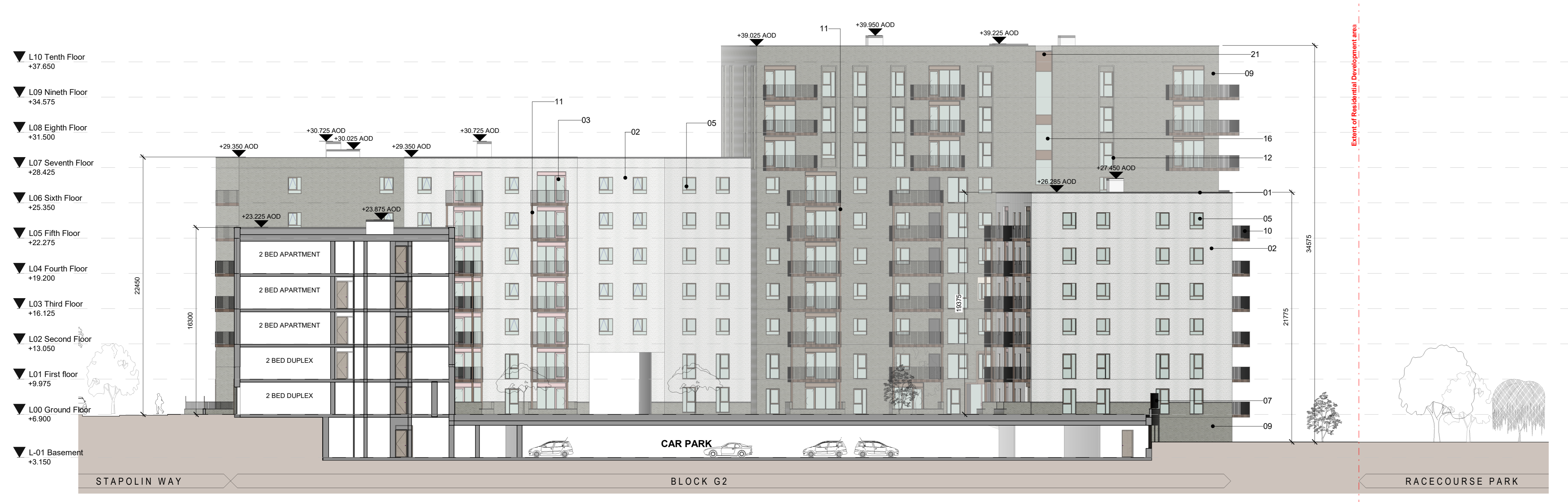
2 SECTION FF 1 : 200
