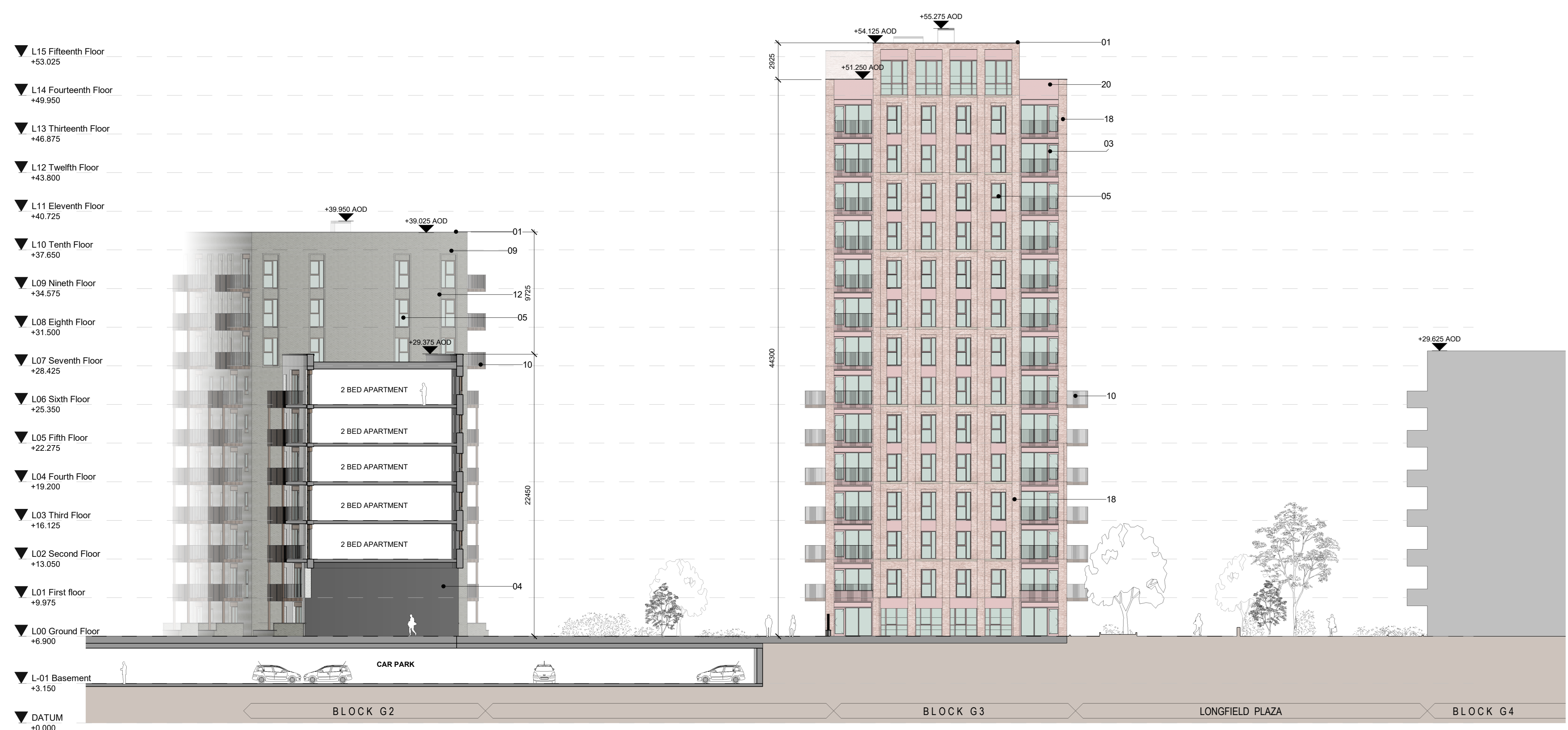
3 SECTION GG 1 : 200
