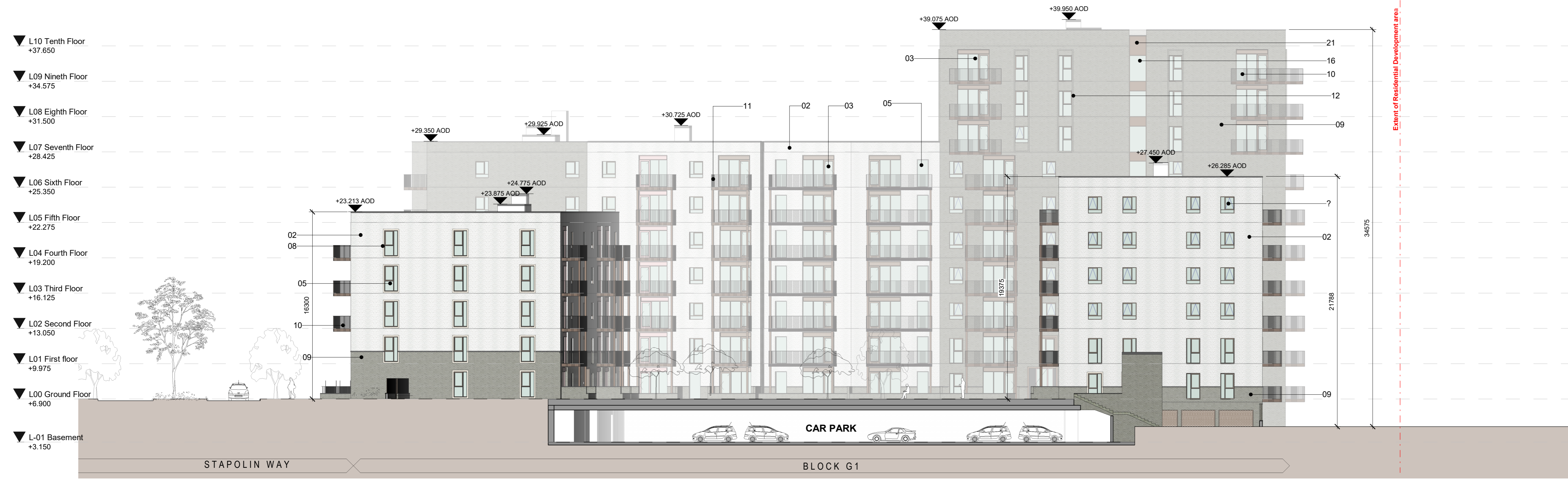
1 SECTION EE 1 : 200
